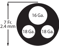
Sección transversal del catéter
