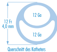
Querschnitt des Katheters
